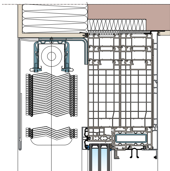
svislý řez prosklenou stěnou Vista s předsaženými raffstory
