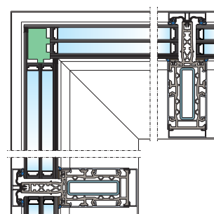
celoprosklený roh
