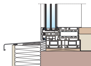
připojení okna zvenku viditelné, zevnitř v jedné rovině s okenním parapetem
