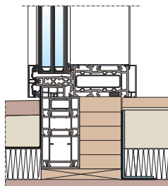
připojení prahu zvenku i zevnitř viditelné
