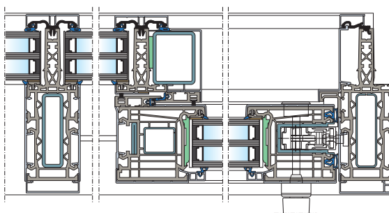
vodorovný řez systému prosklené stěny Vista s integrovanými zvedacími-posuvnými dveřmi
