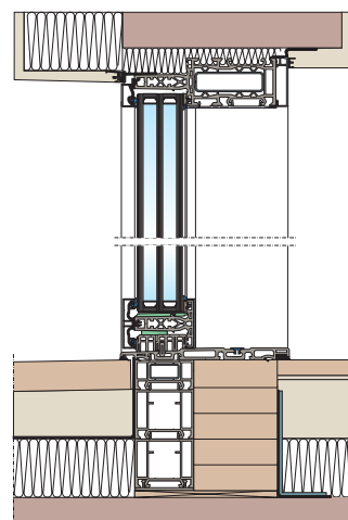
svislý řez C
