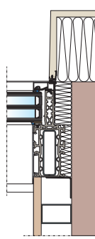
připojení zvenku i zevnitř skryté
