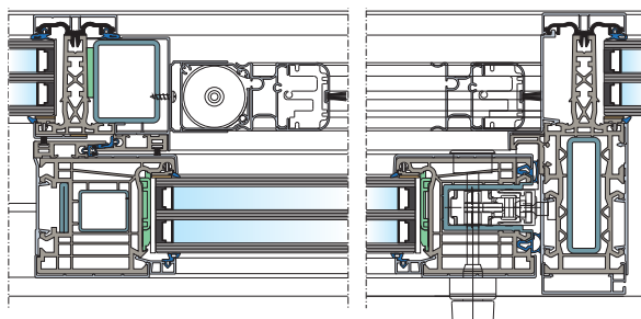
vodorovný řez zvedacími-posuvnými dveřmi se sítí proti hmyzu
