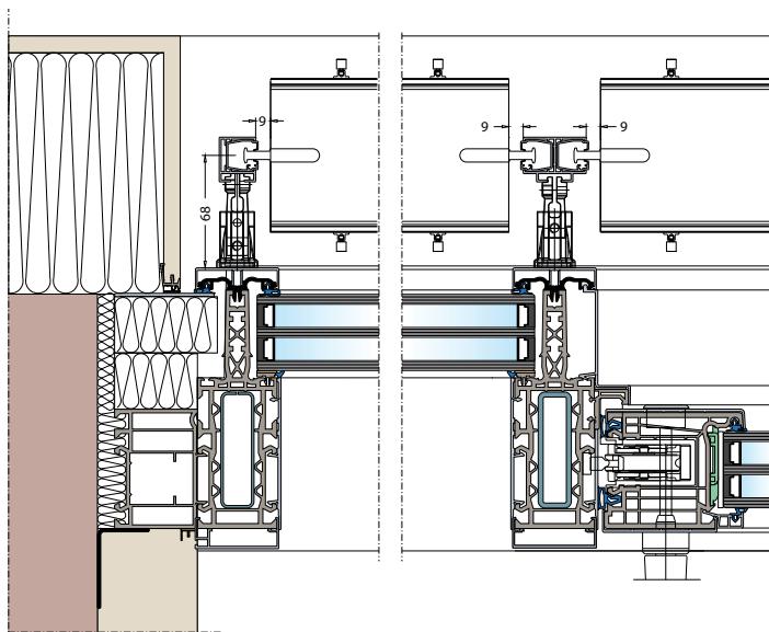
vodorovný řez prosklenou stěnou Vista s předsaženými raffstory
