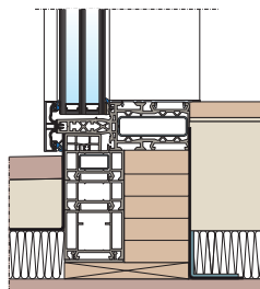
připojení prahu viditelné zvenku, zevnitř v jedné rovině s podlahou
