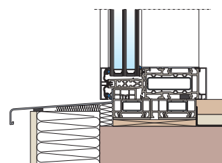
připojení okna zvenku i zevnitř viditelné
