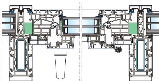
vodorovný řez systému prosklených stěn Vista s vloženým hliníkovým oknem FIN-Project Nova-line
