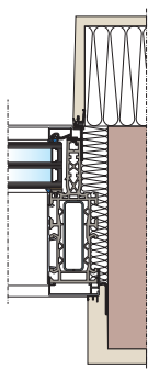
připojení zvenku pod omítku
