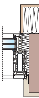
připojení zvenku k fasádním deskám
