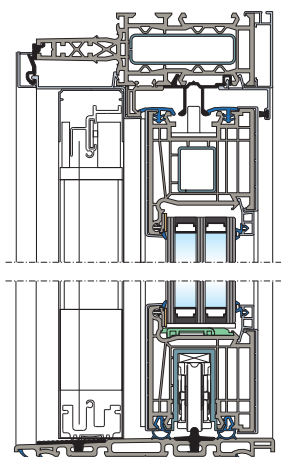
svislý řez zvedacími-posuvnými dveřmi se sítí proti hmyzu
