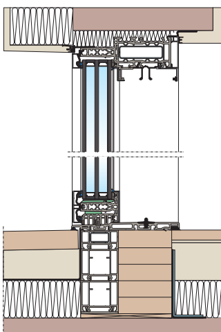
svislý řez B
