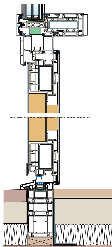
svislý řez prosklenou stěnou Vista s hliníkovými domovními dveřmi
