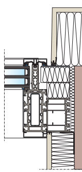
připojení s izolujícím rozšířením
