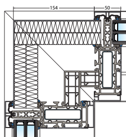
rohové napojení 90°
