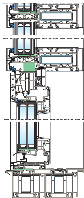
svislý řez s otvírávámi-sklopnými dveřmi FIN-Project Nova-line s plochým prahem
