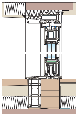
svislý řez A
