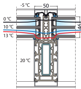
tepelně izolující konstrukce sloupku s hodnotou U_f 1,1 \text{ W/m}^2\text{K}
