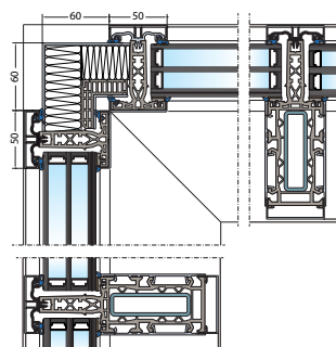
štíhlé rohové napojení 90°
