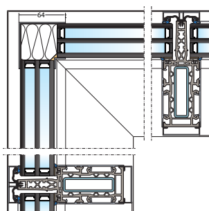
prosklený roh 90°
